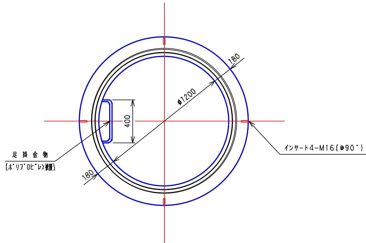
平面図 S = 1/20
