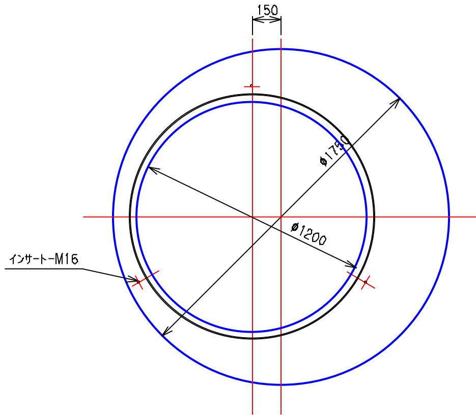
平面図 S = 1 / 20
